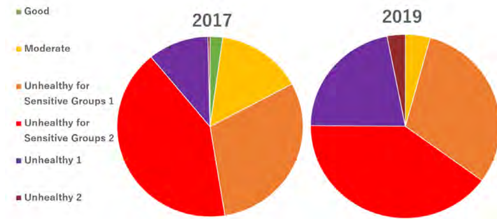
図1 一年間の各大気汚染レベルの一日の平均比率
