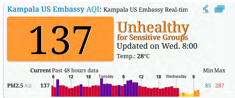
図2 3月18日水曜日午前8時から48時間の大气汚染レベル
